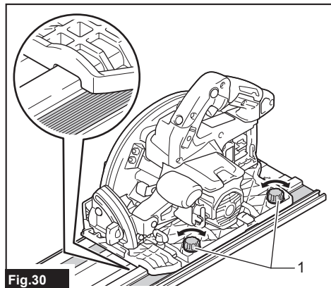
Fig.30 ► 1. Tornillos de ajuste
